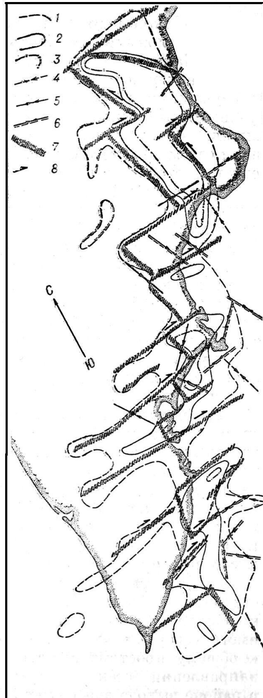
Рис.8. Плотность очагов землетрясений Камчатки. Глубина гипоцентров более 100 км [Эрлих, 1973]. Сводка по [Токарев и др., 1968, 1970, 1970а, Федотов и др., 1967, 1970, Аверьянова, 1968]. Изолинии плотности эпицентров для квадратов со стороной 25 км, где отмечено 1 – одно, 2 – три, 3 – 5 и более землетрясений. Векторы сжатия по [Zobin, 1979], 4 – с глубиной очага 60-70
