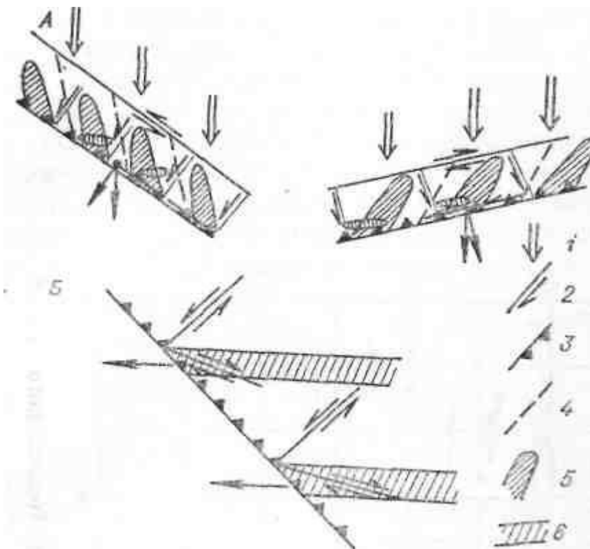
Рис. 9. Схема воздействия движений по сейсмофокальной зоне на структуры коры. [Эрлих, 1973].
