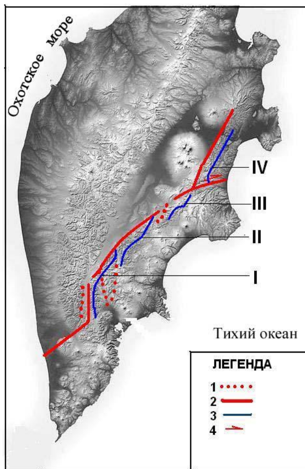
Рис. 23. Морфоструктуры Восточного хребта, предположительно образованные растяжением, ориентированным вдоль основного разлома. Рисунок выполнен В. И. Белоусовым по проекту Э. Эрлиха.
