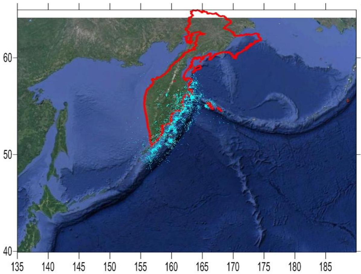
Рис.2. Эпицентры землетрясений в период 1990-1994 годов. ( K_s = 5-18 , h = 0-700 км).
