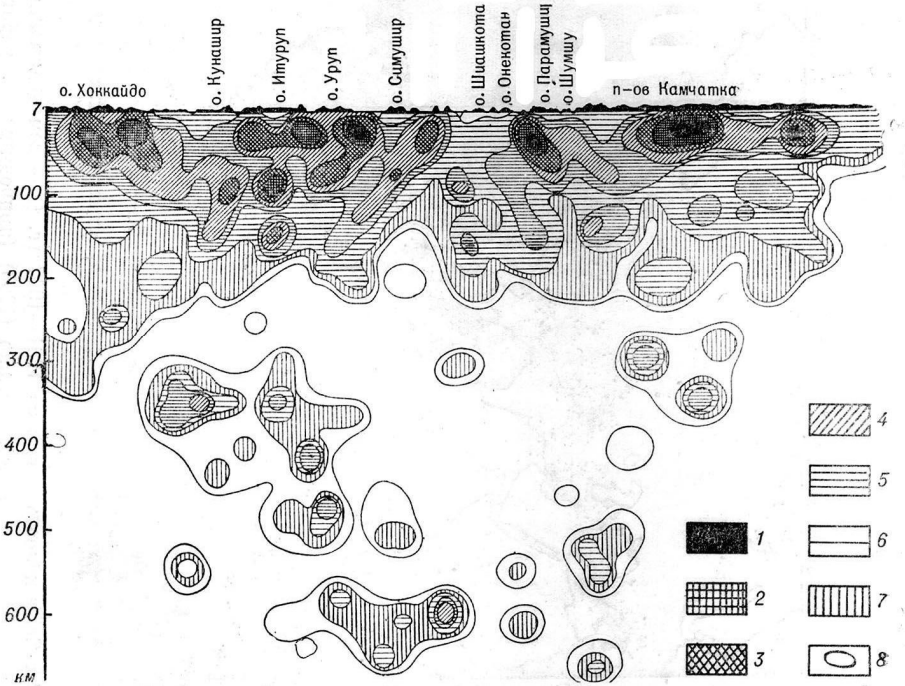
Рис.11. Продольный разрез Курило-Камчатской сейсмофокальной зоны [Аверьянова, 1968]. Области, в пределах которых сумма энергии, выделившейся в очагах землетрясений за
