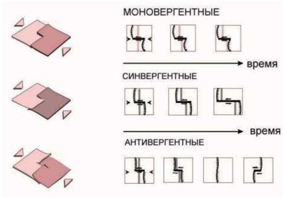
Рис. 13. Общая схема трансформов [Тевелев, 2003].
