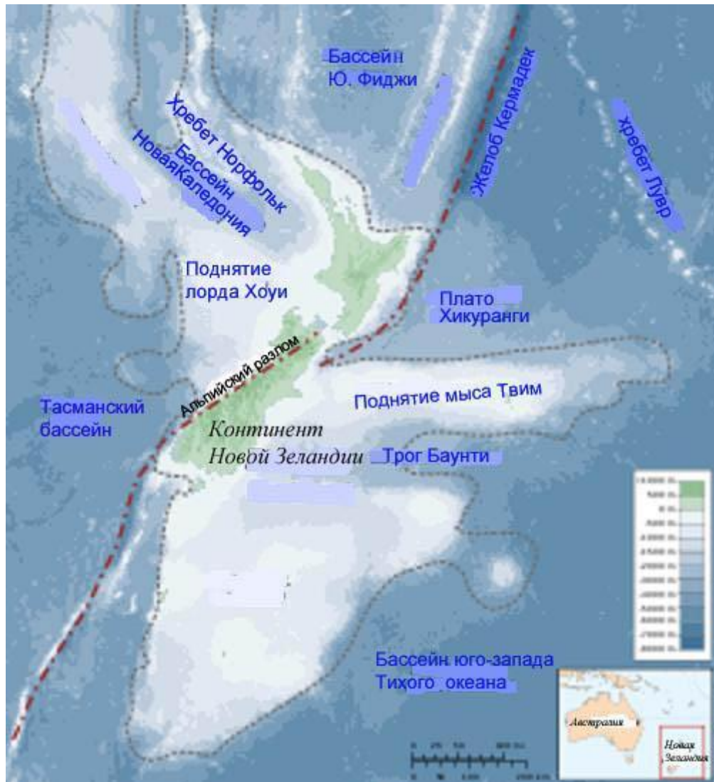
Рис. 4. Кососекущий характер Альпийского разлома Новой Зеландии [Wellman, 1944].
