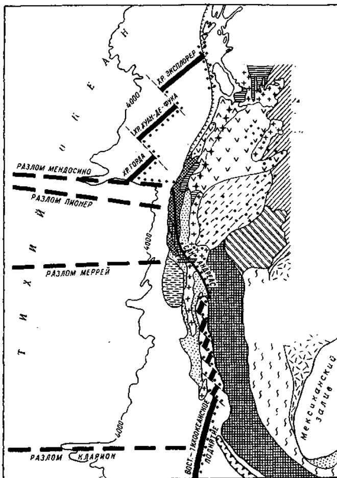
Рис. 25. Тектоническая схема рифтовых долин и трансформных разломов северо-восточной части Тихого океана [из Гончаров, Телицкий, Фролова, 2005].
