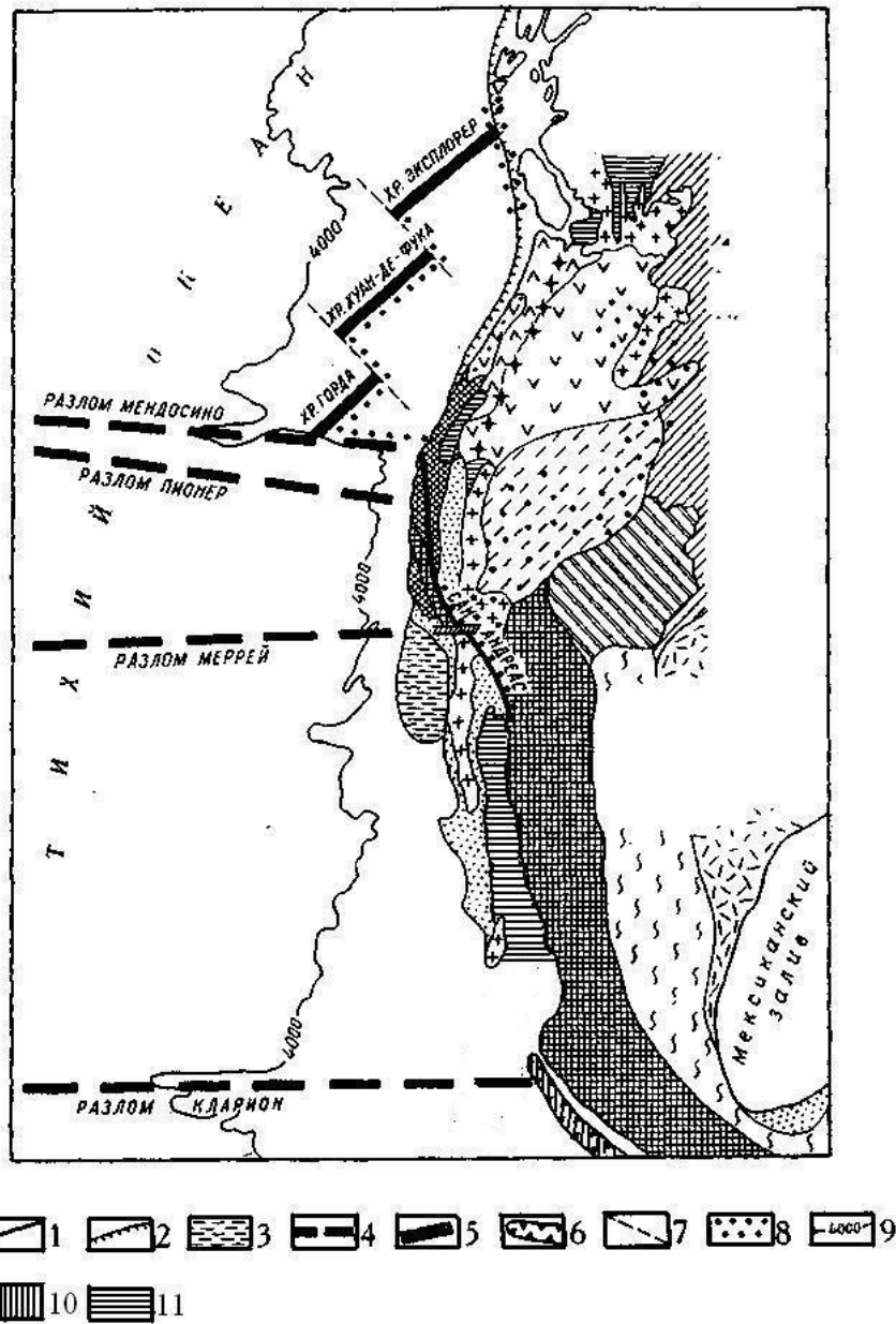
Рис. 26. Соотношение Центрально-Американского желоба, грабена Калифорнийского залива и разлома Сан-Андреас [упрощено из Гончаров, Телицкий, Фролова, 2005].
