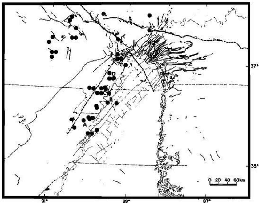
Рис.29. Эпицентры и разломы вдоль Нью-Мадридской сейсмической зоны. В центральной части США. По [Sykes, 1978]. Сравнение с рис. 22 показывает параллельность эпицентральной зоны
