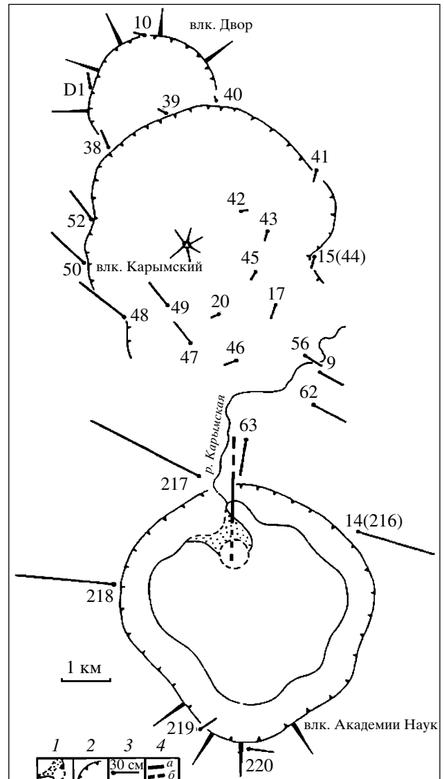
Рис. 2. Горизонтальные деформации земной поверхности вблизи вулкана Карымский и вокруг Карымского озера после извержений 01–02.01.1996 г. за период от 1989, 1990–1995 гг. до 05.1996 г., вычисленные относительно пункта 7 и направления 7–8 (рис. 1). 1 – кратер в озере и новый полуостров, образовавшийся при извержении; 2 – границы кальдер вулканов Двор, Карымский и Академии Наук; 3 – направление и величина горизонтальных подвижек пунктов, их масштаб и номер пункта; 4 – открытая трещина растяжения (а), предполагаемое продолжение трещины (б).
