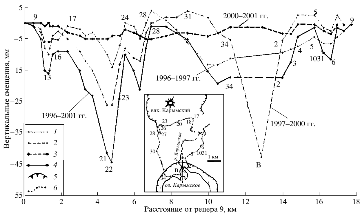
Рис. 8. Вертикальные движения вдоль нивелирного профиля в периоды: 1 – 1996–1997 гг.; 2 – 1997–2000 гг.; 3 – 2000–2001 гг.; 4 – 1996–2001 гг. Буквой В обозначен репер, заложенный на новом полуострове. Услов. обозн. см. на рис. 2 и 6.
