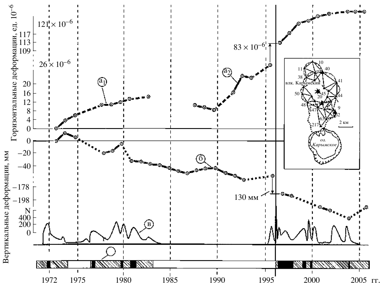
Рис. 9. Сопоставление подвижек земной поверхности с активностью вулкана в 1972–2005 гг. a 1 – среднее значение изменений длин линий в ед. 10^{-6} в линейно-угловой сети вокруг конуса вулкана, ограниченной пунктами 48-50-38-11-10-40-41-44-9-47; a 2 – то же на участке, ограниченной пунктами 20-45-44-9-62-63-217-47; б – вертикальные смещения репера 20 относительно пункта 40 с 1972 по 1996 гг. и далее относительно репера 9 с 1996 по 2005 гг.; в – ежесуточное число взрывных землетрясений (тип N_4 по [18]); г – активность вулкана: I – фазы покоя; II – фазы эксплозивного извержения; III – фазы эффузивно-эксплозивного извержения [18]. На вставке показана схема линейно-угловой сети геодезических пунктов и линия нивелирования.
