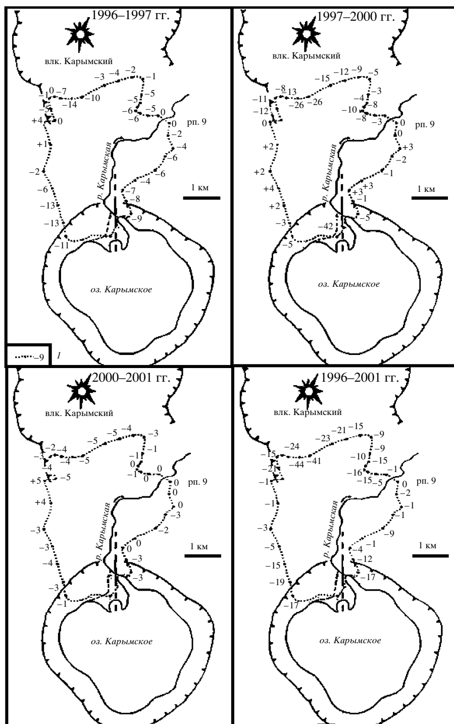
Рис. 7. Вертикальные движения реперов в мм в разные периоды. 1 – линия нивелирования и вертикальное движение репера. Услов.обозн. см. на рис. 2.
