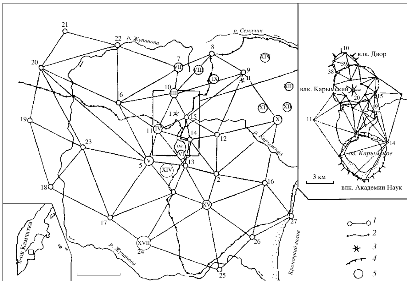
Рис. 1. Схема геодезических работ в Карымском вулканическом центре. 1 – стороны линейно-угловой триангуляции; 2 – линии высокоточного нивелирования; 3 – действующие стратовулканы: I – Карымский; II – Малый Семячик; 4 – кальдеры вулканов Карымский, Академии Наук и Двор (на врезке); 5 – потухшие вулканы Карымской группы (цифры в кружках): III – Двор, IV – Разлзтый, V – Крайний, VI – Академии Наук и Однобокий, VII – Соболиный, VIII – Ступенчатый бастион, IX – Сухой, X – Прибрежный Южный, XI – Стена, XII – Прибрежный Северный, XIII – Массивный, XIV – Березовый, XV – Дитмара, XVI – Белянкина, XVII – Жупановские Востряки.
