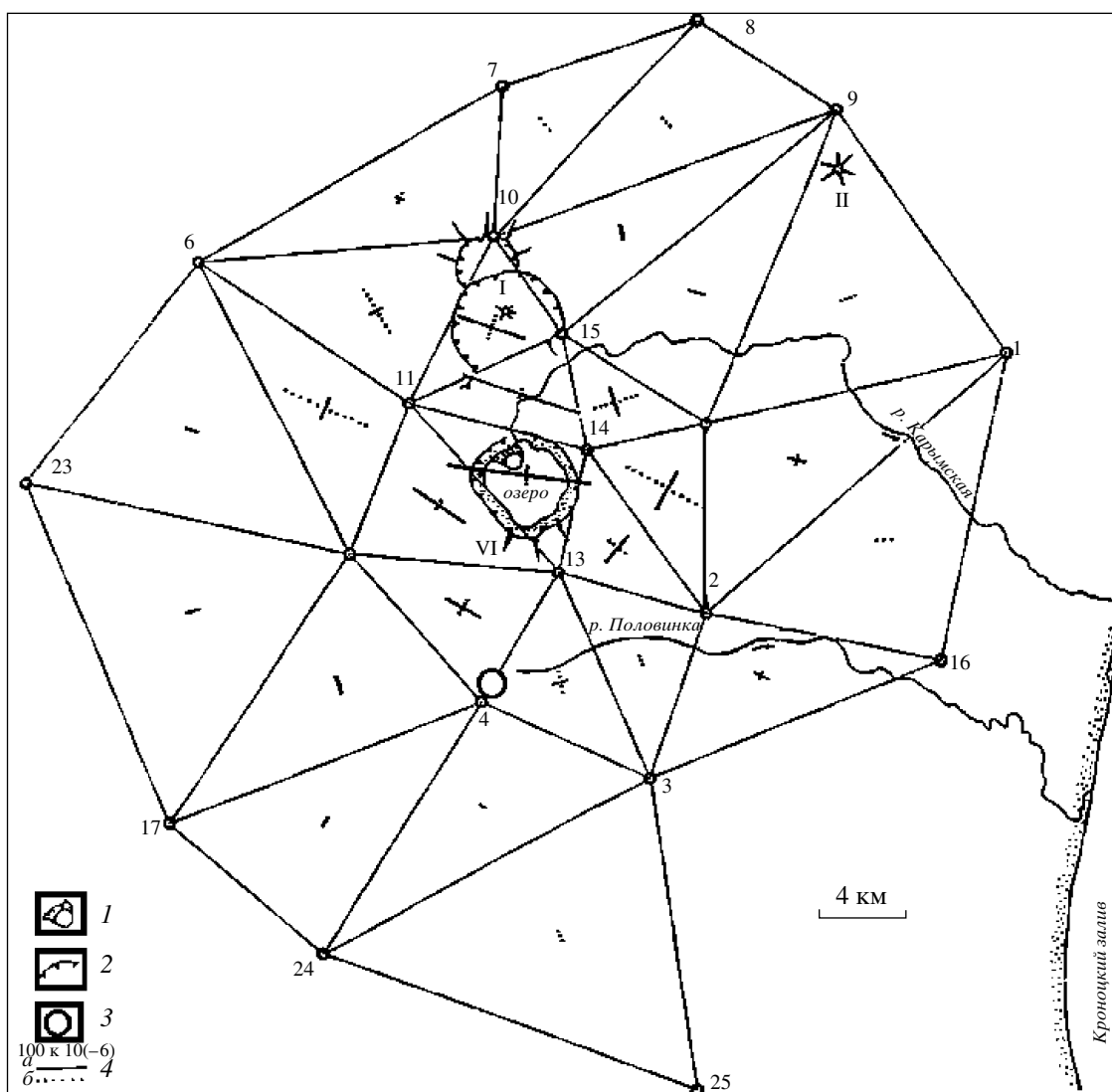
Рис. 3. Направления главных осей плоской деформации растяжения-сжатия и их величины в Карымском вулканическом центре после извержений 01–02.01.1996 г. в период от 1988 до 1996–2000 гг. (в 1996, 1997, 1999 и 2000 гг. были получены данные на всей площади, которые объединены в одну эпоху). 1 – кратер подводного извержения в кальдере Академии Наук и новый полуостров, образовавшийся при извержении; 2 – границы кальдер; 3 – эпицентр главного землетрясения 01.01.1996 г., M = 6.9; 4 – масштаб плоской деформации: а – растяжение, б – сжатие. Вулканы: I – Карымский, II – Малый Семейчик, VI – Академии Наук.
