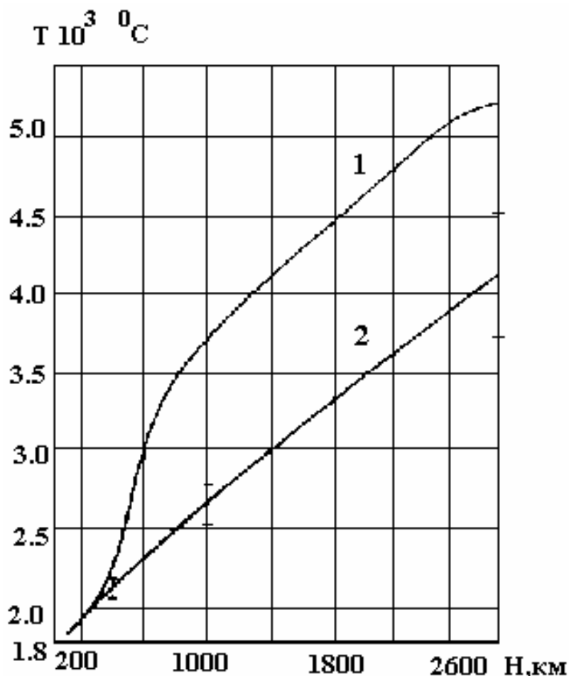
Рис. 8.4. Кривые плавления в оболочке Земли в диапазоне глубин от 100 км до границы ядра, в предположении, что T_{m0} ( H = 100 км) = 1800^{\circ}\text{C} . Вертикальные линии на кривых показывают границы неопределенности. Видно, что температура на границе ядра, по-видимому, не может превышать 5000^{\circ}\text{C} [Магницкий, 1965; с. 33].
