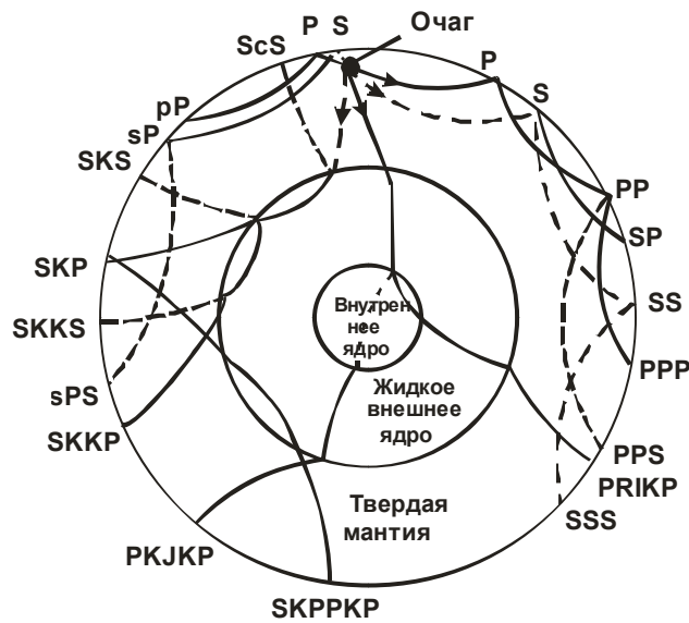
Рис. 4.5. Сейсмические лучи, соответствующие годографам на рис.4.4, по Буллину. _____ лучи P, - - - лучи S.
