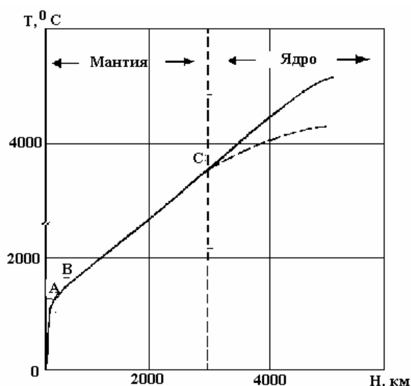
Рис. 8.6. Вероятное распределение температур внутри Земли [Магницкий, 1965, с. 38]
