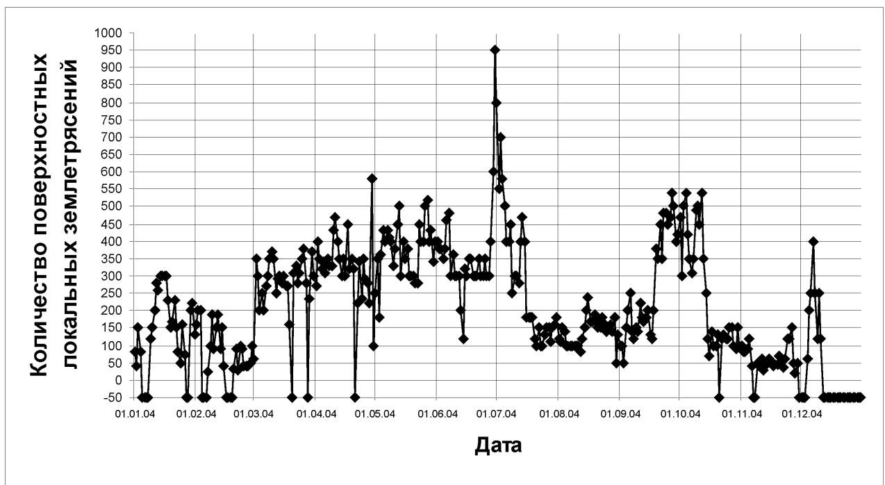
Рис. 12. Сейсмичность вулкана Карымский в 2004 г. по данным сейсмостанции «KRY». Значение «-50» означает отсутствие данных.
