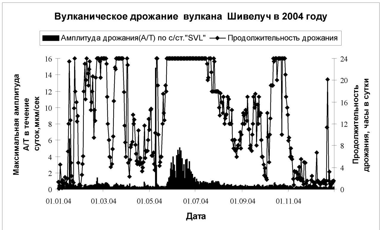
Рис. 9. Вулканическое дрожание вулкана Шивелуч в 2004 г.
