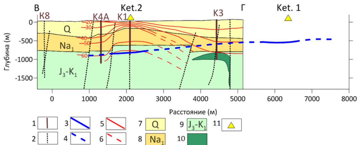
Рис. 3. Совмещенные с геологическим разрезом В-Г [7] полученные данные МТЗ. 1 – скважины Кеткинского геотермального месторождения; 2 – тектонические нарушения, установленные дешифрированием и геофизическими работами, и частично заверенные бурением; 3, 4 – граница, выделенная по данным МТЗ, пунктиром – предполагаемая граница; 5, 6 – изотермы; 7 – нерасчлененная тоща рыхлых четвертичных отложений; 8 – аллейская серия верхнемиоценового-плиоценового возраста; 9 – верхняя юра – нижний мел; 10 – габбродиориты; 11 – пункты МТЗ.
