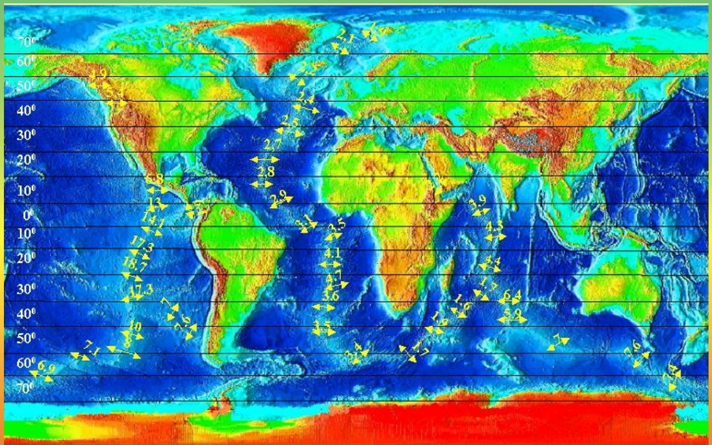
Иллюстрация к статье Кузикас О.В. “Объемы и особенности ....” Рис. 1. Карта рассчитанных скоростей спрединга срединно-океанических хребтов (см/год). Основа карты по http://www.ngdc.noaa.gov/mgg/ .
